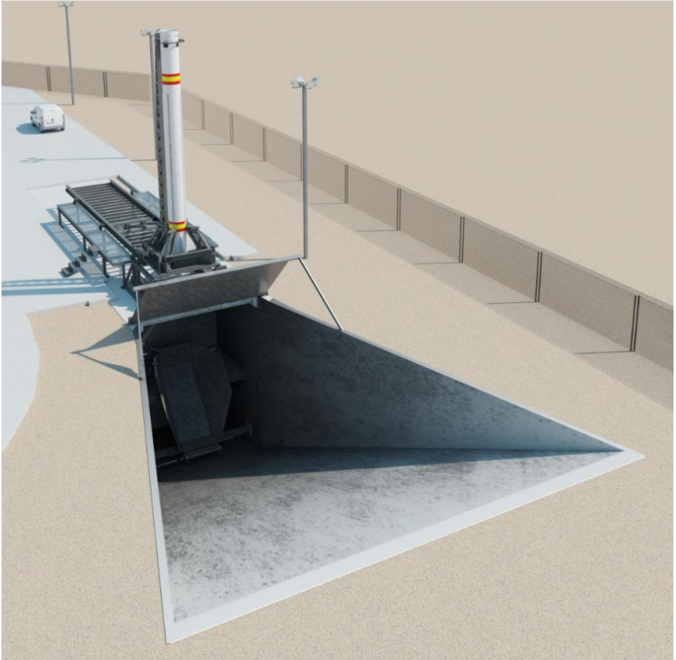
Imagen 2. Banco de ensayos T2 de las instalaciones de PLD Space en el aeropuerto de Teruel
